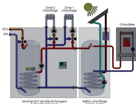
SOLAR COMBIPAQ
